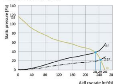
Kennlinien Statischer Druck
