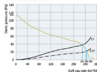
Kennlinien Statischer Druck
