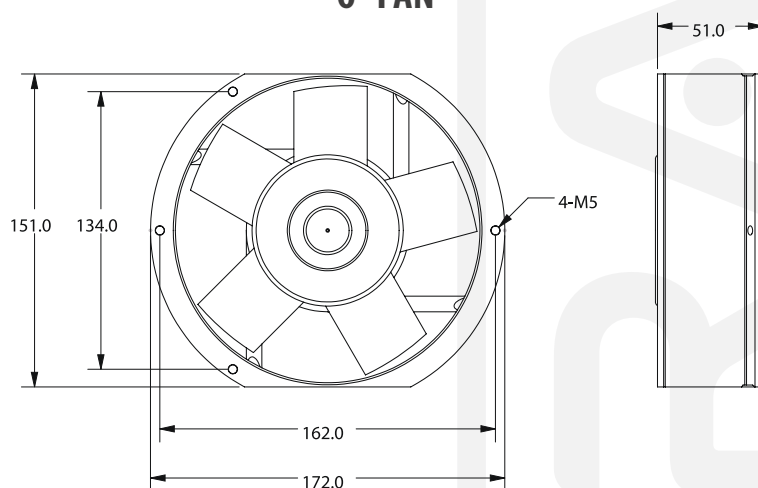
6" FAN
