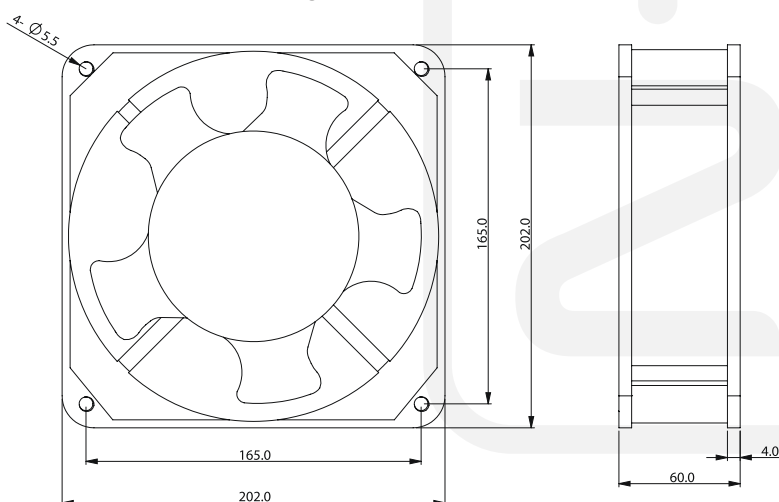
8" FAN
