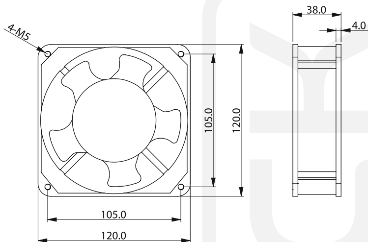
4" FAN
